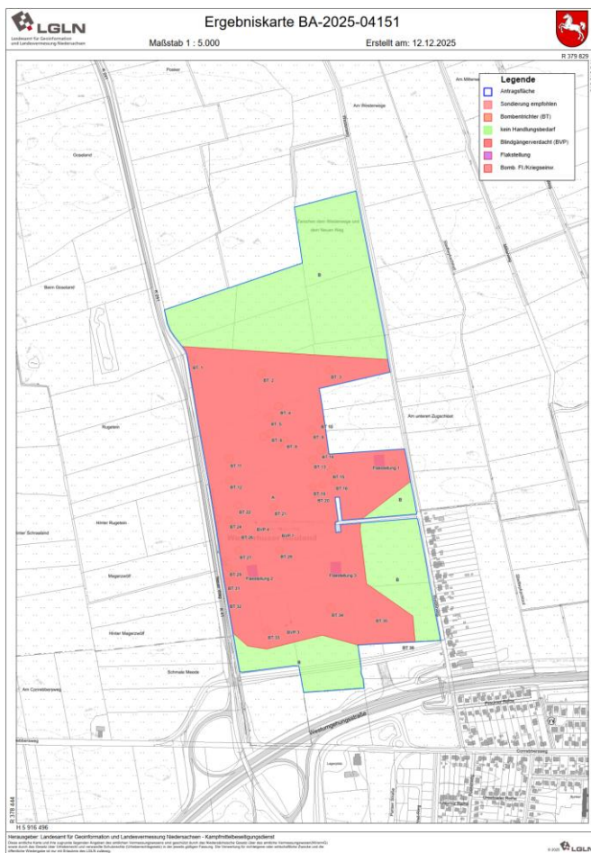
Abbildung 7: Luftbildauswertung, Ergebniskarte 12.12.2025
